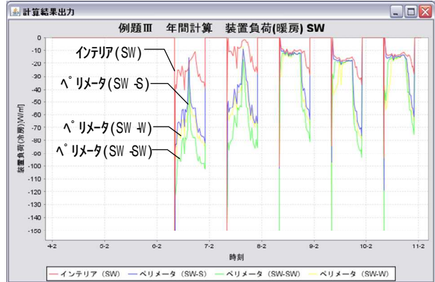
図 2.2.3-5 代表週の装置負荷変動
