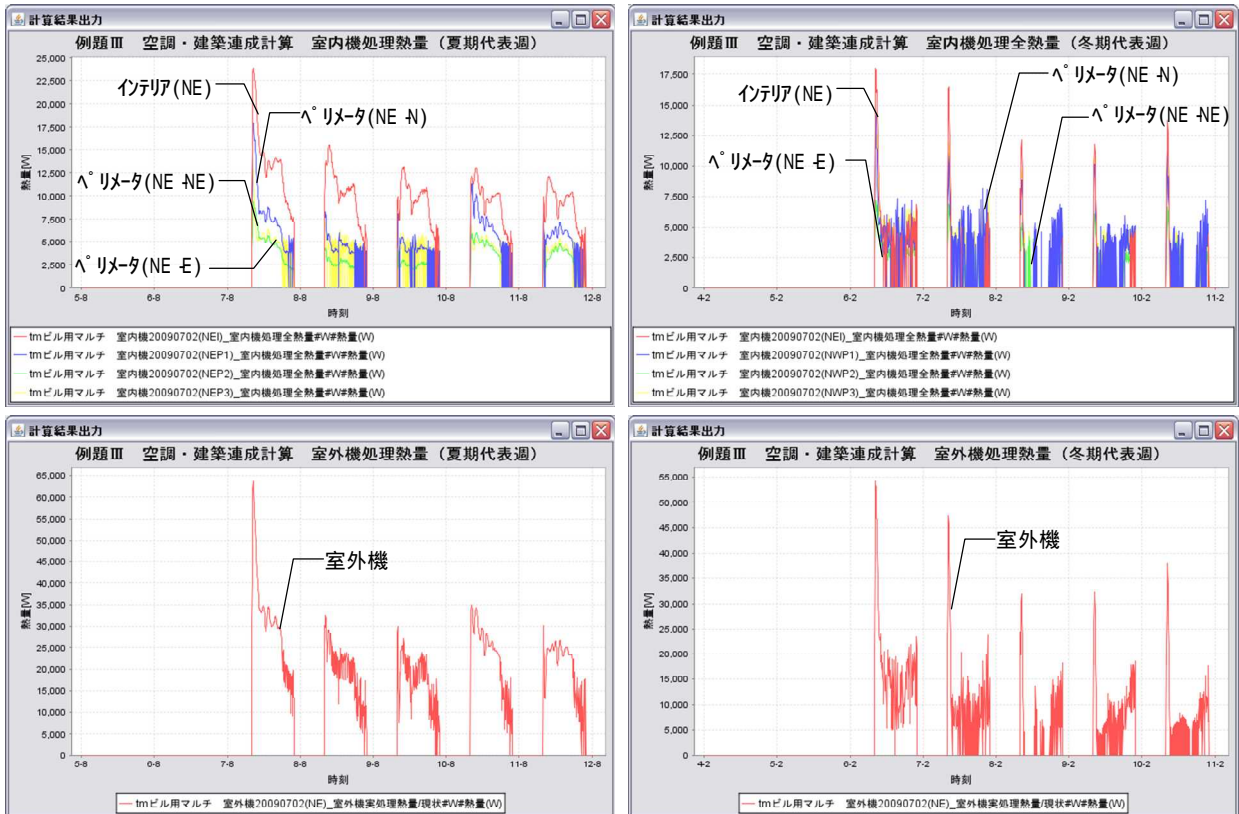
図 2.3.2-11 代表週の処理熱量
