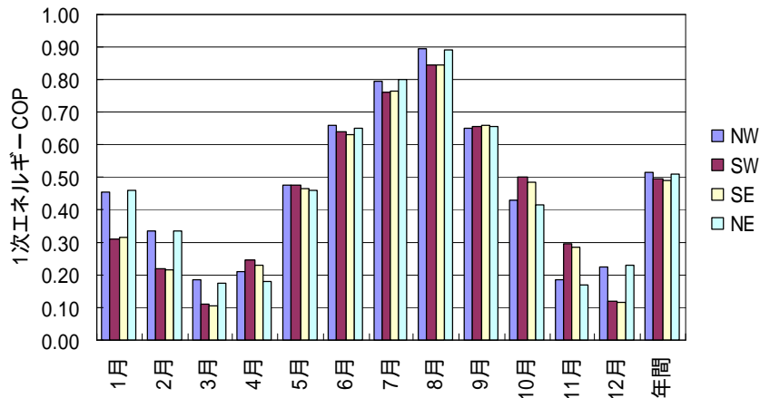
図 2.3.2-15 月別システム COP (室内機 + 室外機)
