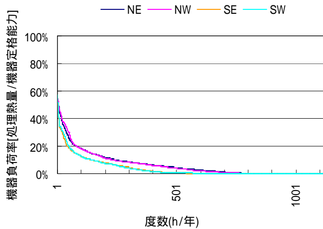
図 2.3.2-19 機器負荷率のデューリング線図
