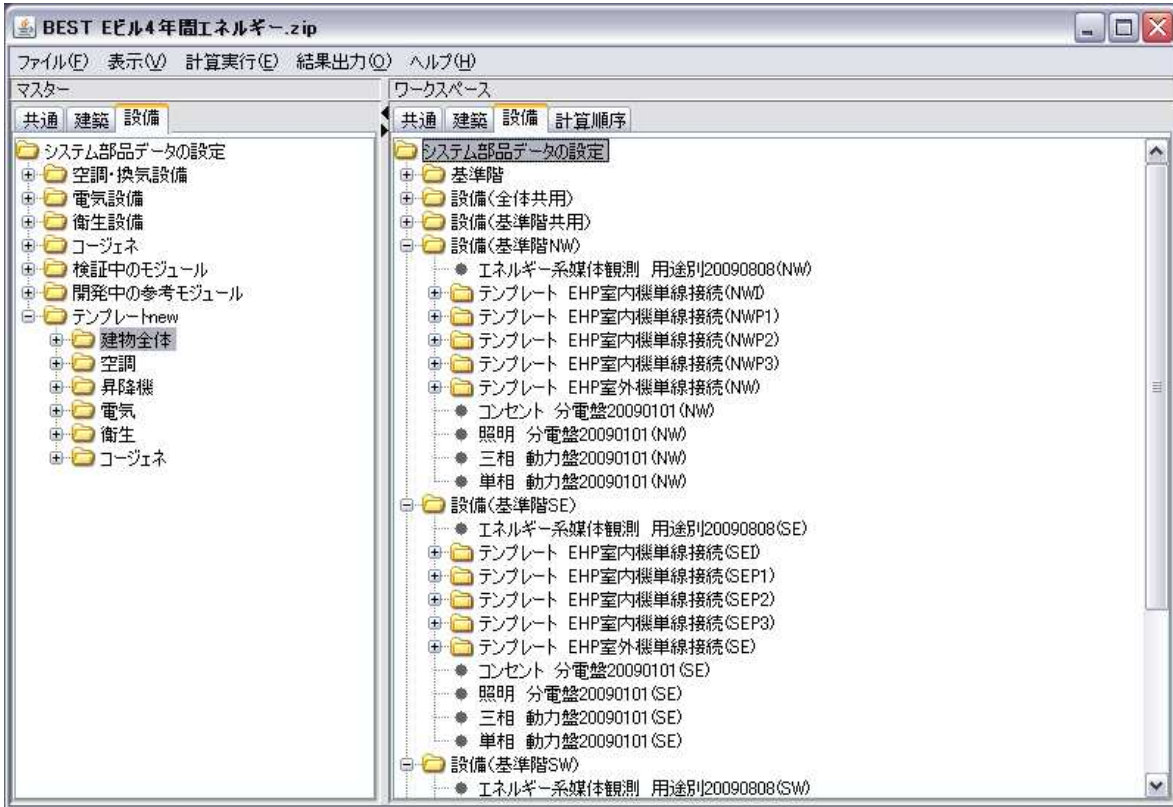
図 2.3.1-1 空調設備のモジュール構成
