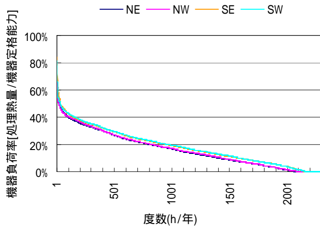
図 2.3.2-17 機器負荷率のデューリング線図
