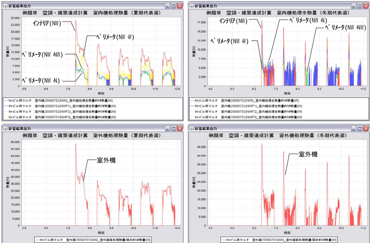
図 2.3.2-2 代表週の処理熱量
