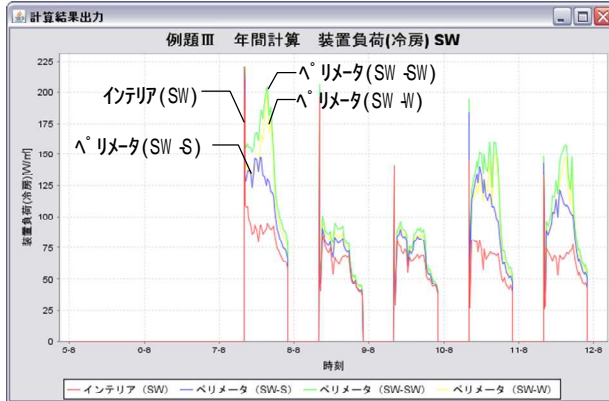
図 2.2.3-5 代表週の装置負荷変動
